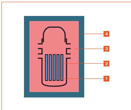
Principiální schéma ochranných bariér jaderné elektrárny
